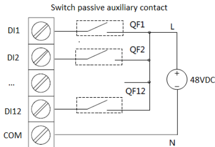
Figure 2-30 DI Wiring
